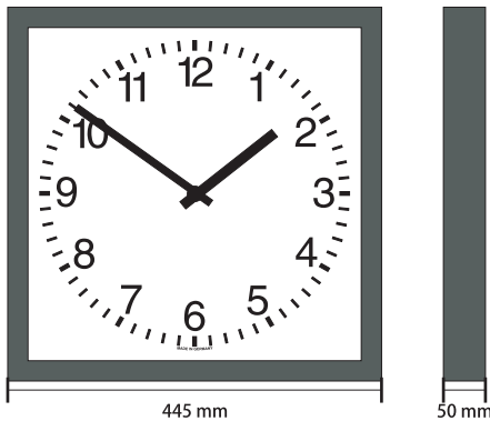
Aussenabmessungen des Gehäuses H x B x T: 445 mm x 445 mm x 50 mm
