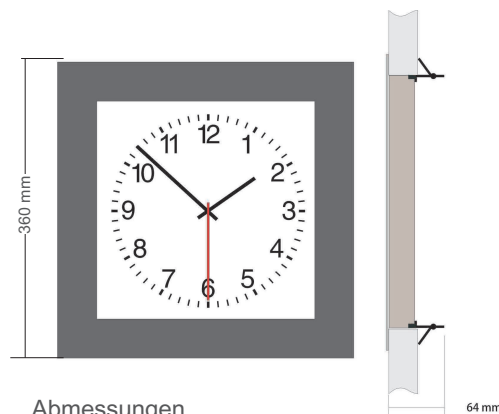
Abmessungen
